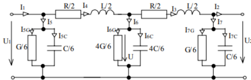
Obrázok 12 - Steinmetzov článok
