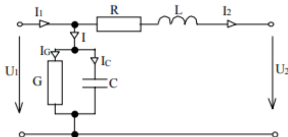
Obrázok 9 - \Gamma článok
