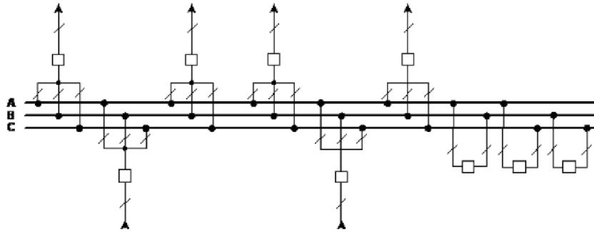
Obrázok 5 – trojitý systém prípojnic
