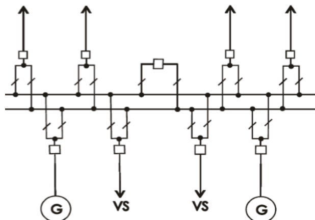
Obrázok 3 - viacsystémová prípojnica
