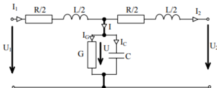
Obrázok 11 - T článok
