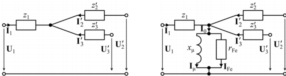
Obrázok 14 - náhradná schéma 3vinutového TR
