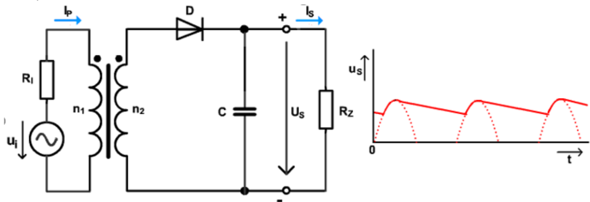
Obrázok 17 - jednocestný usmerňovač
