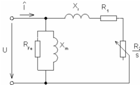
Obrázok 24 - náhradná schéma asynchrónneho generátora
