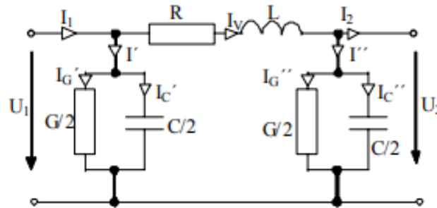
Obrázok 10 - \Pi článok
