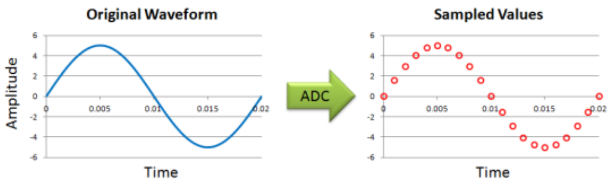
Obrázok 52 - schéma vzorkovania
