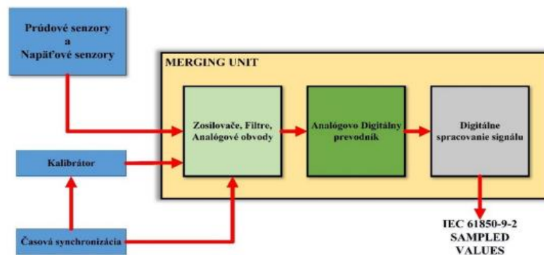
Obrázok 51 - merging unit
