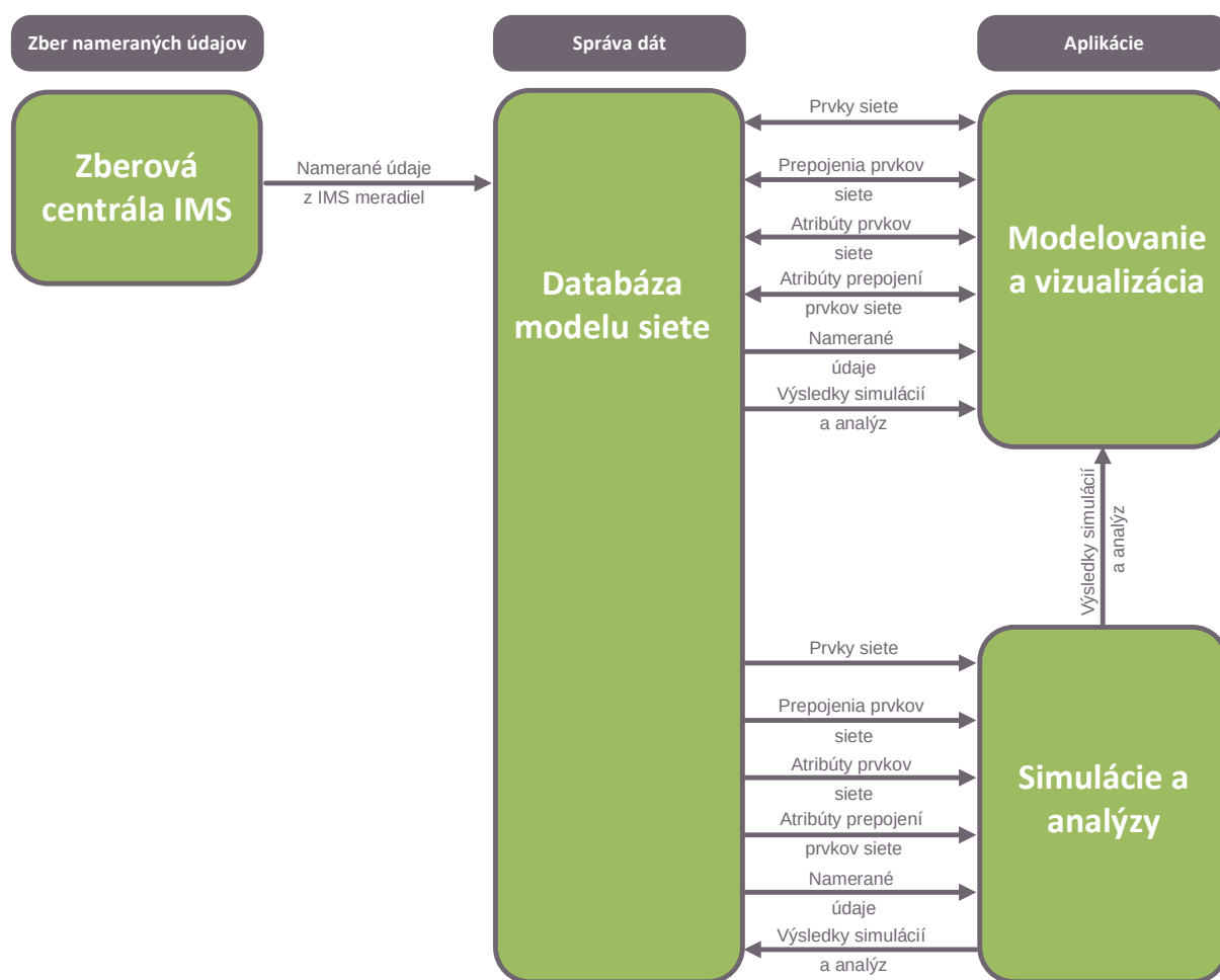
Obrázok 32 - Interné rozhrania
